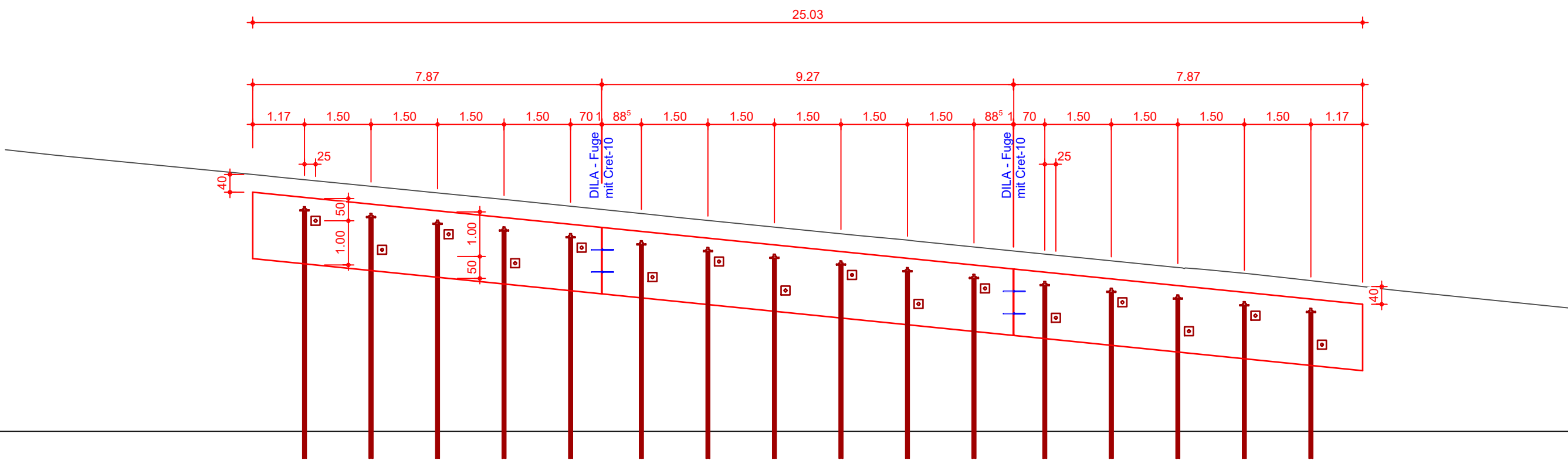
Längsschnitt, 1:100
