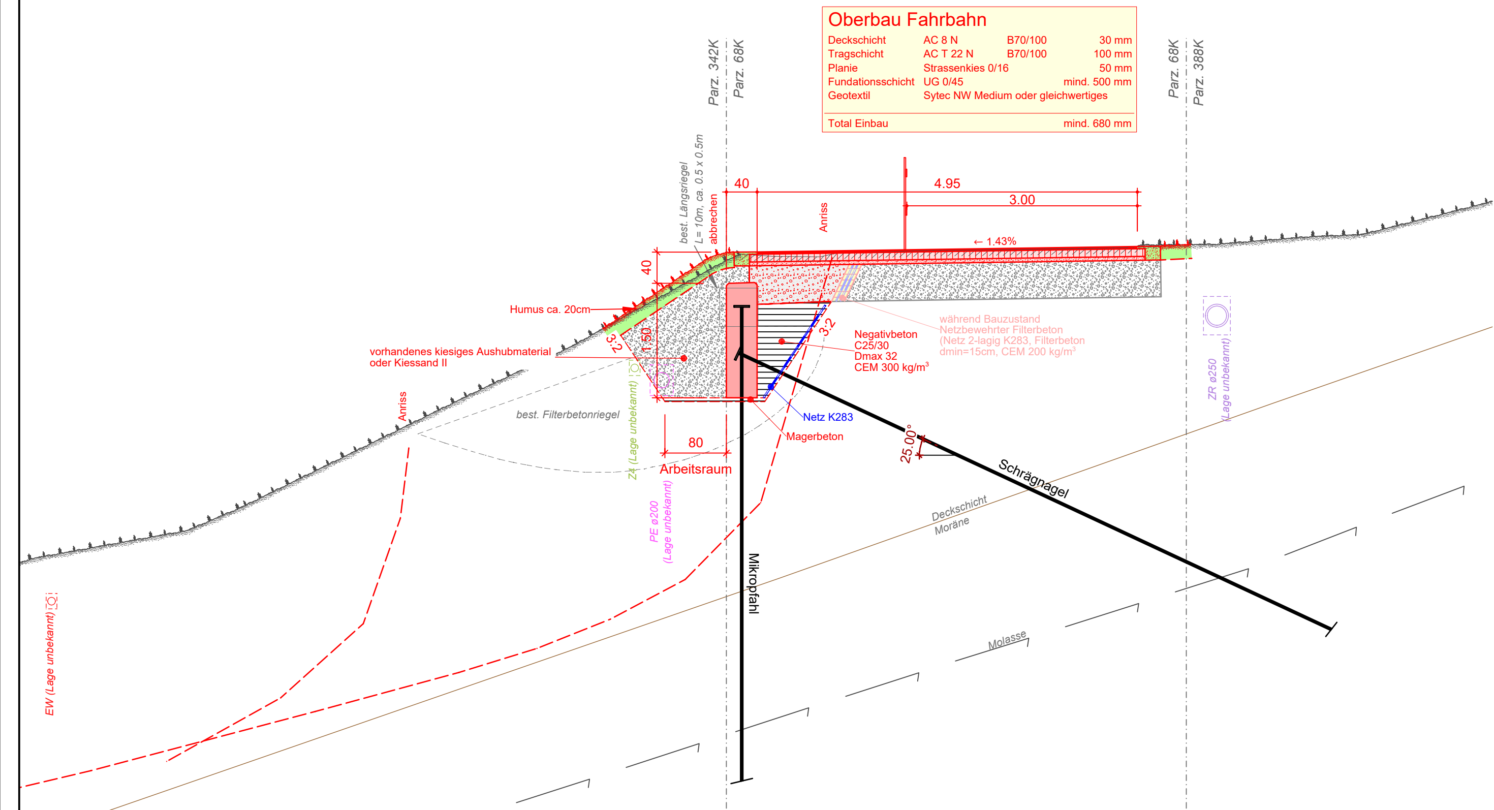
Normalprofil, 1:50
